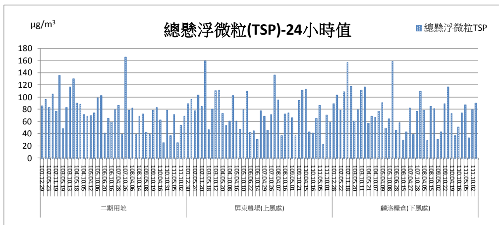
圖 2.1-1TSP 各測點 24 小時監測結果比較圖
