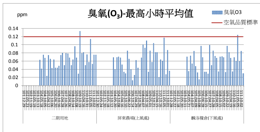
圖 2.1-14 臭氧各測點最高小時平均值監測結果比較圖
