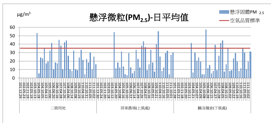
圖 2.1-15 PM 2.5 各測點日平均監測結果比較圖
