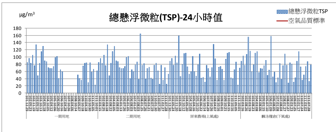
圖 2.1-1TSP 各測點 24 小時監測結果比較圖
