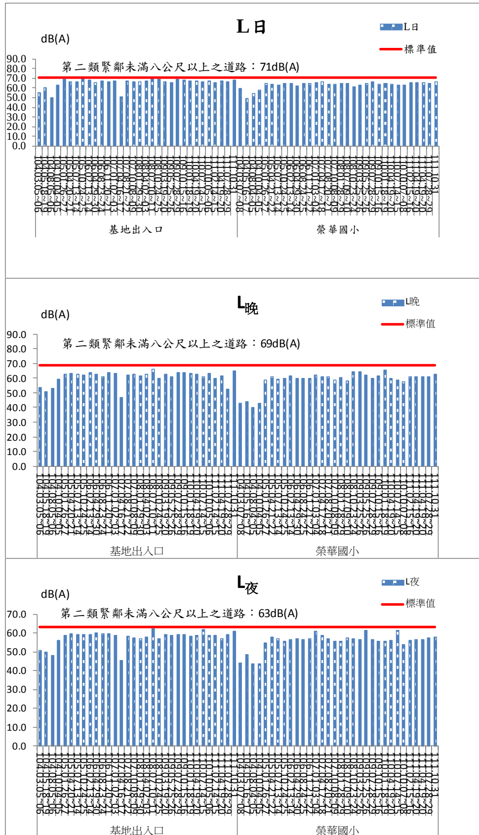
圖 2.2-1 基地出入口及榮華國小噪音監測結果比較圖
