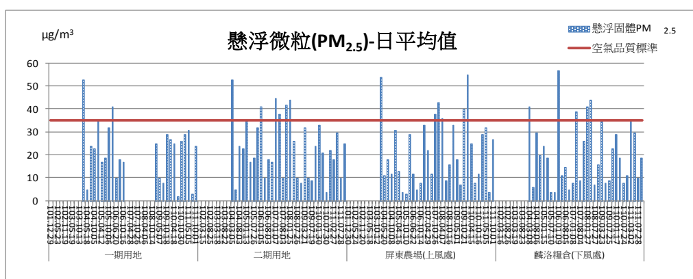
圖 2.1-15 PM 2.5 各測點日平均監測結果比較圖
