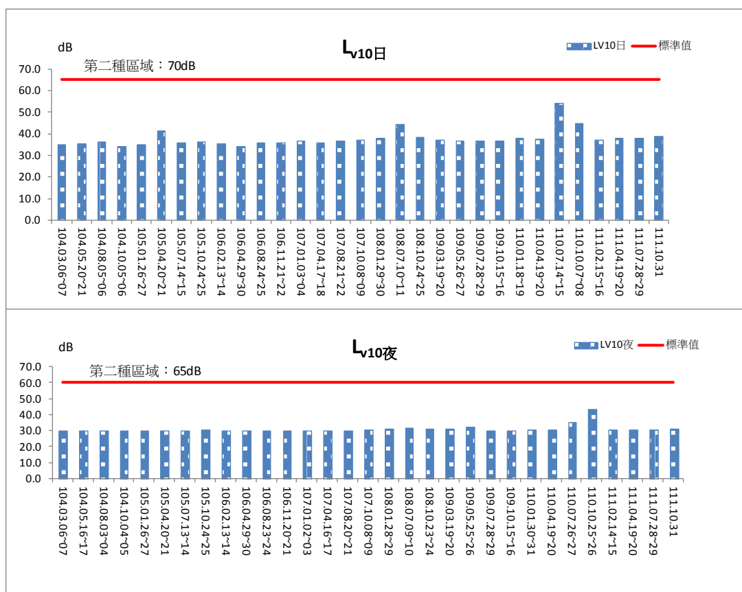
圖 2.2-4 屏 37 縣道與省道台 1 線交接處振動監測結果比較圖
