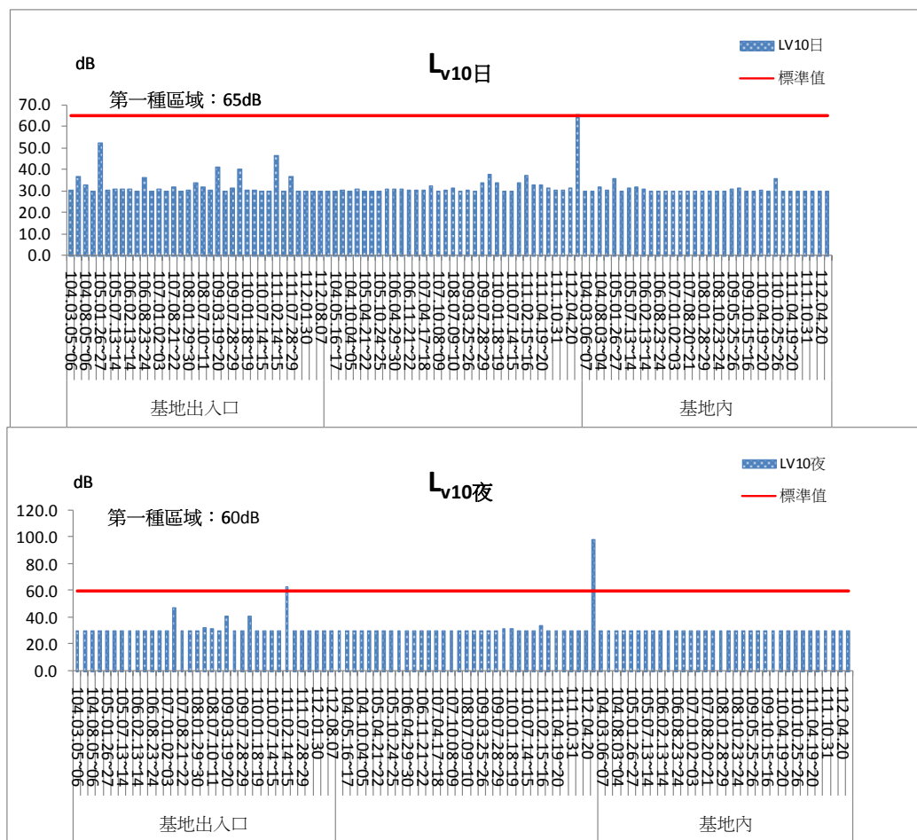
圖 2.2-3 基地出入口、榮華國小及基地內振動監測結果比較圖
