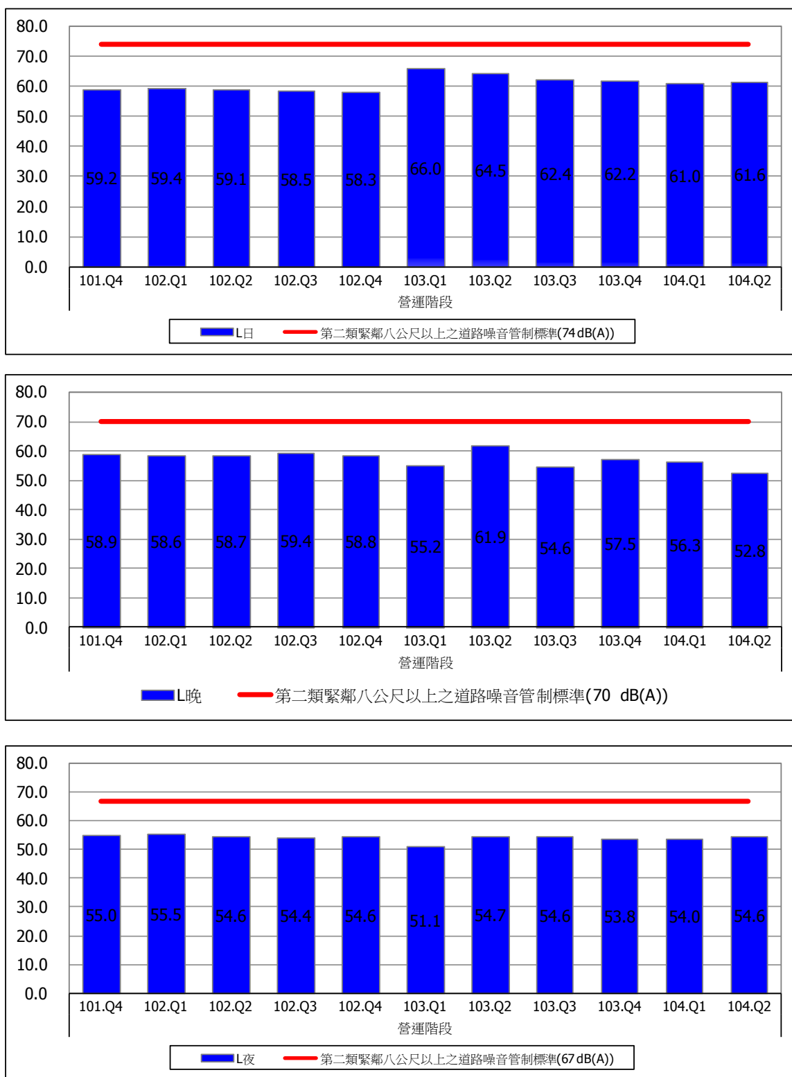
圖 2.2-1 基地出入口噪音監測結果比較圖
