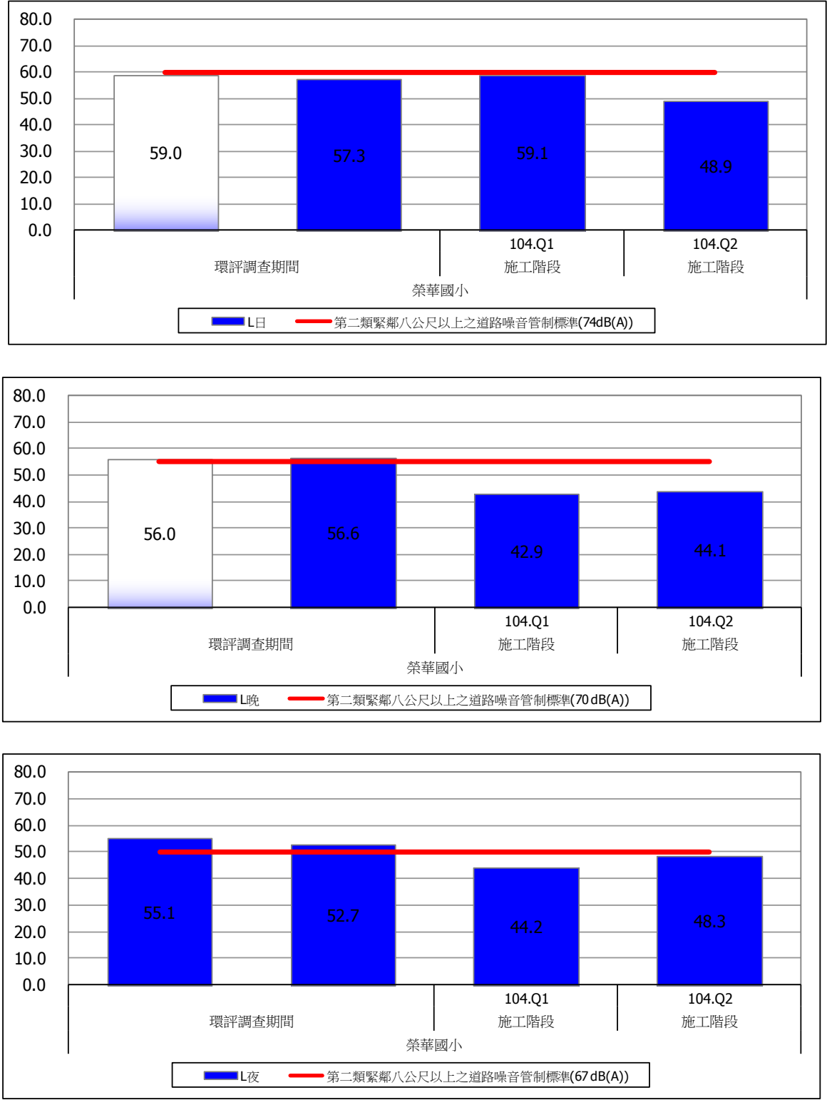
圖 2.2-3 榮華國小噪音監測結果比較圖
