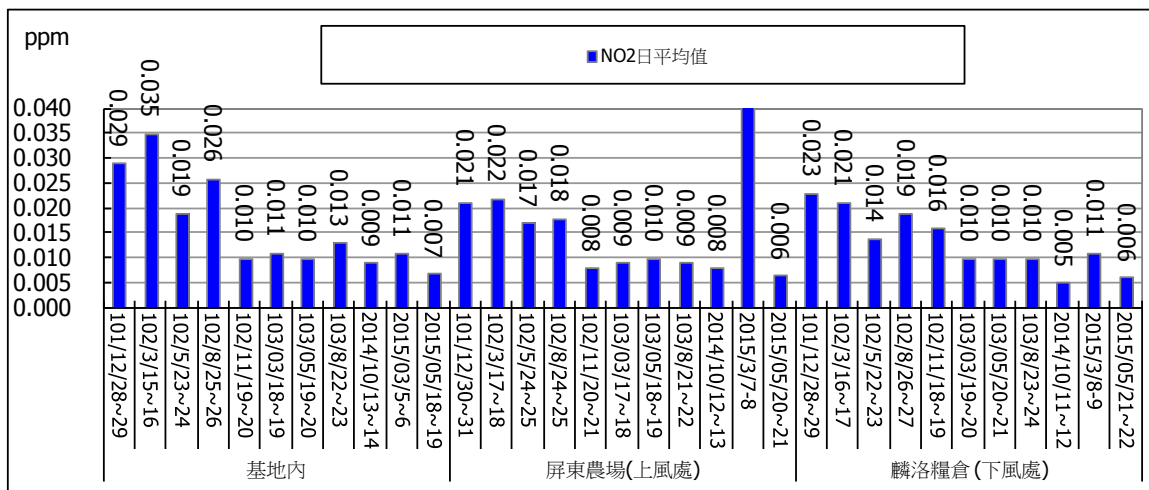
圖 2.1-5 一氧化氮各測點日平均值及點最高小時平均值監測結果比較圖
