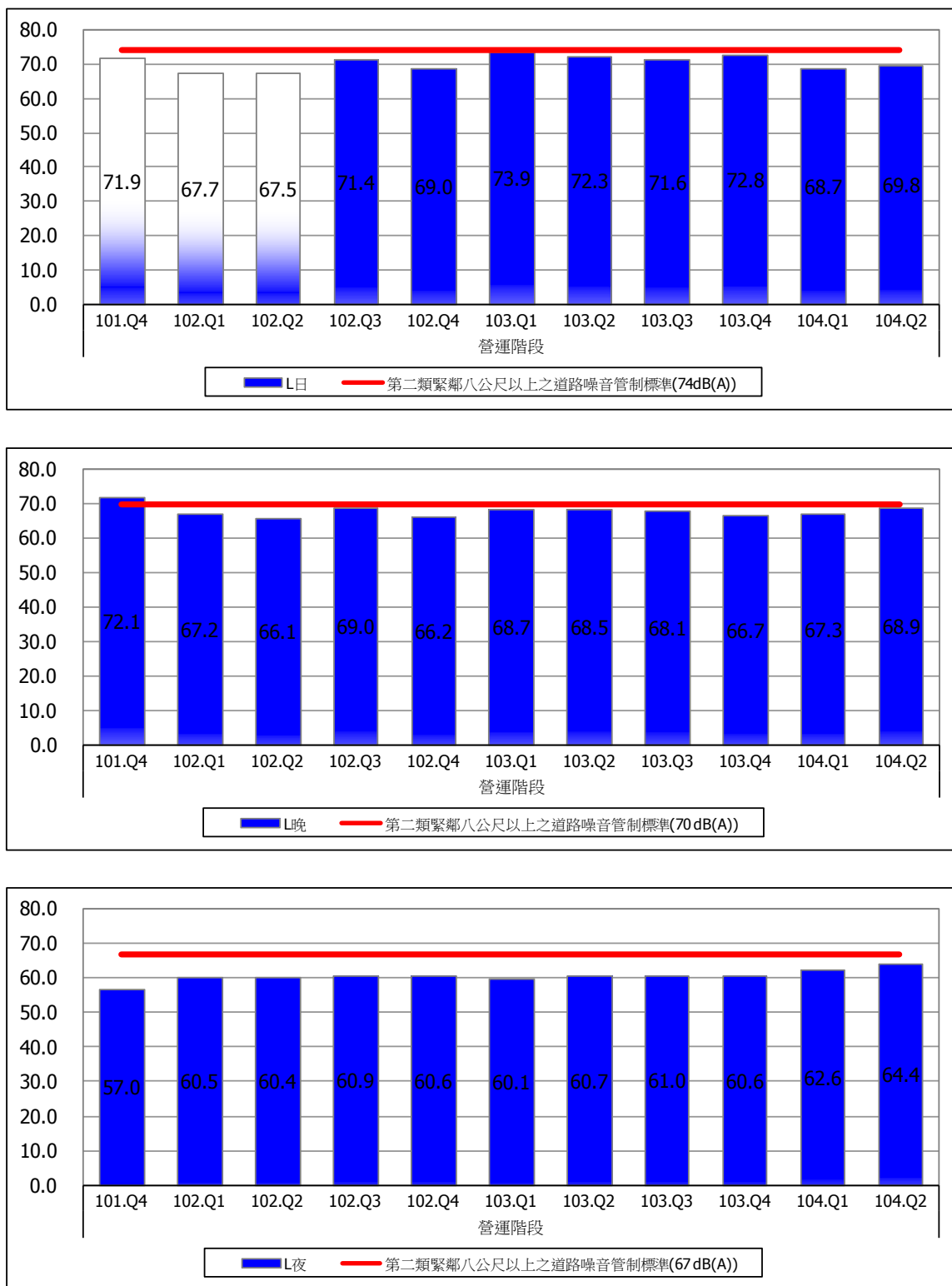
圖 2.2-2 屏 37 鄉道與台 1 省道交接處噪音監測結果比較圖
