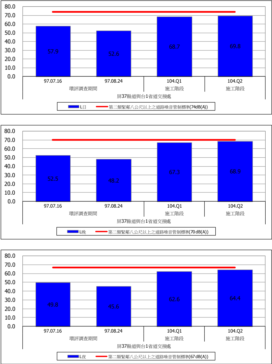
圖 2.2-4 屏 37 與台 1 省道噪音監測結果比較圖
