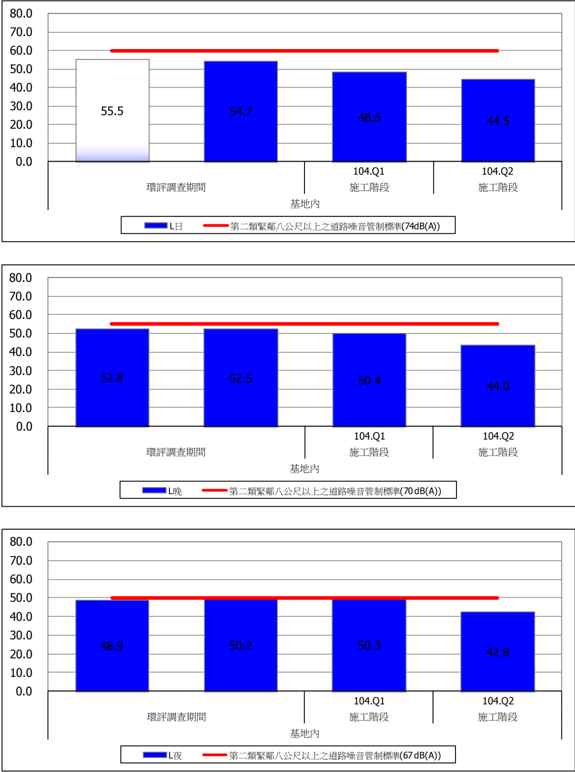
圖 2.2-2 基地內噪音監測結果比較圖
