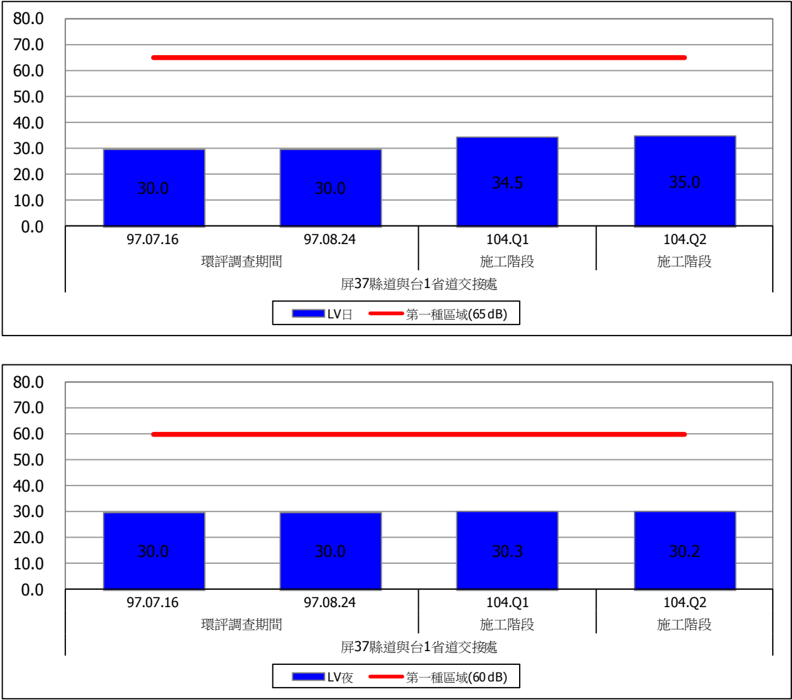
圖 2.2-8 屏 37 與台 1 省道振動監測結果比較圖
