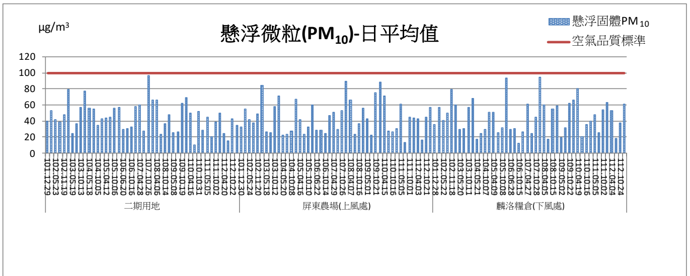
圖 2.1-2PM 10 各測點日平均值監測結果比較圖
