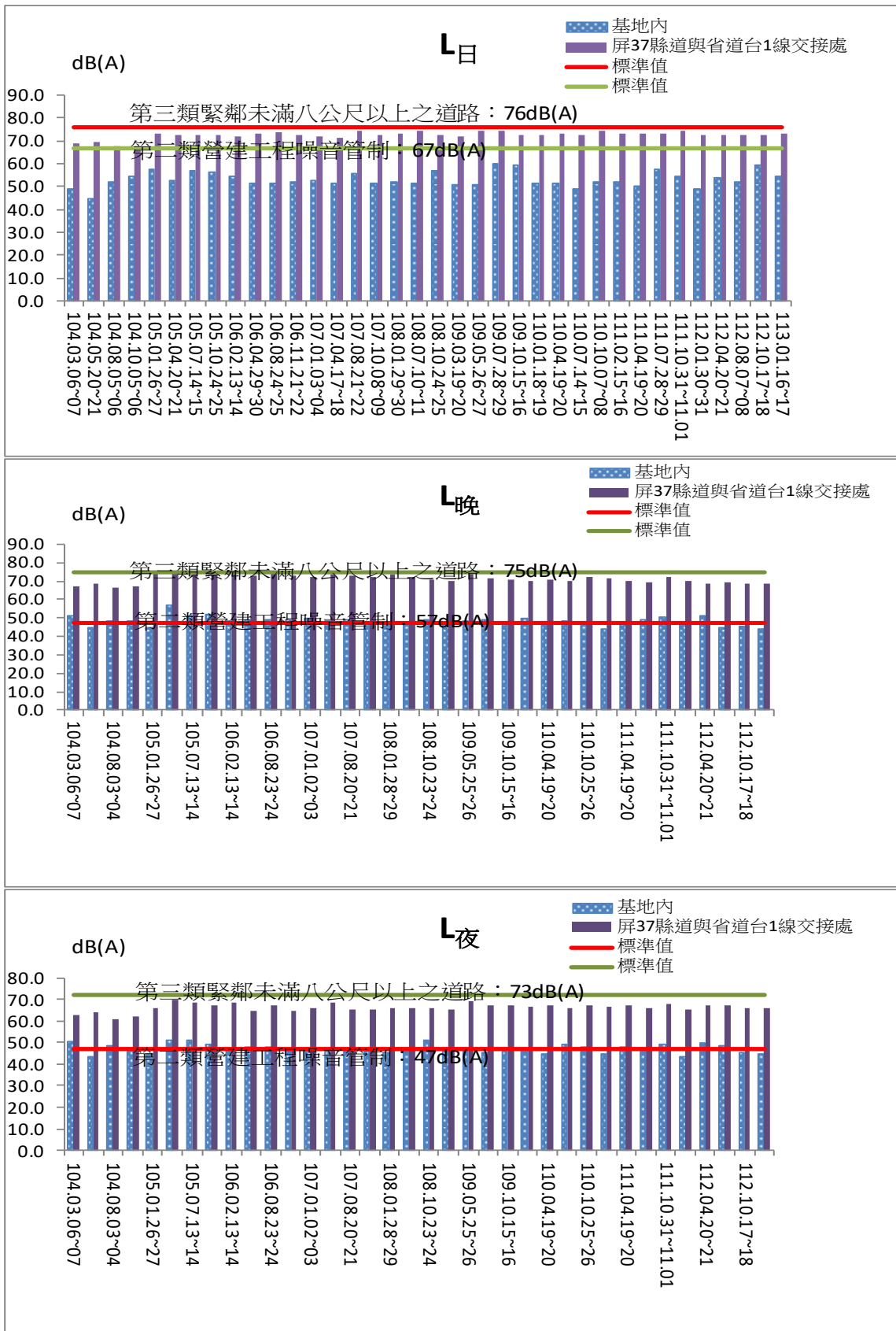
圖 2.2-2 基地內及屏 37 縣道與省道台 1 線交接處噪音監測結果比較圖
