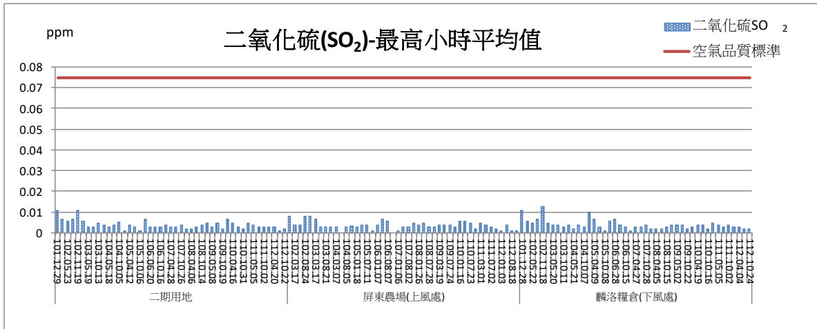
圖 2.1-4 二氧化硫各測點最高小時平均值監測結果比較圖
