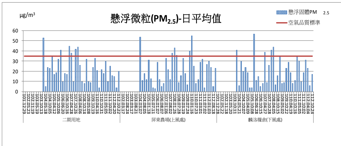
圖 2.1-15 PM 2.5 各測點日平均監測結果比較圖
