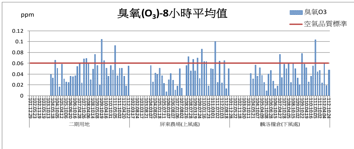
圖 2.1-13 臭氧各測點最高八小時平均值監測結果比較圖
