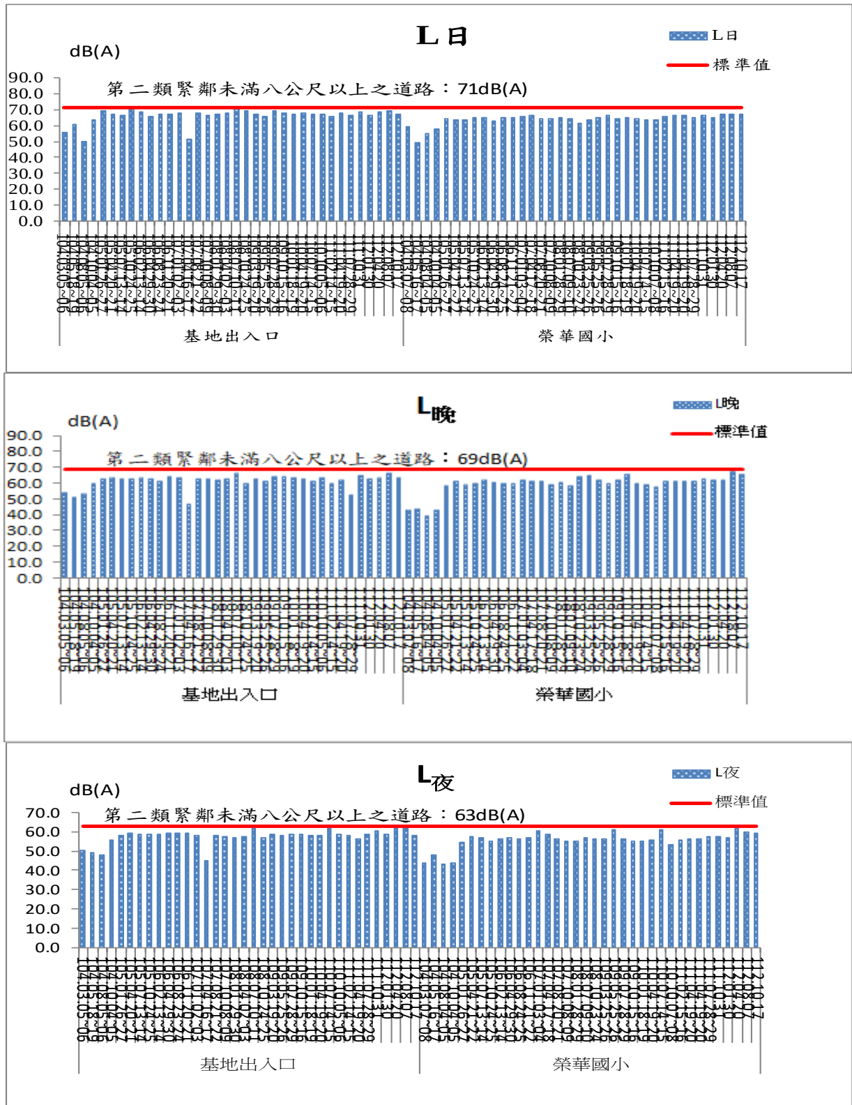
圖 2.2-1 基地出入口及榮華國小噪音監測結果比較圖
