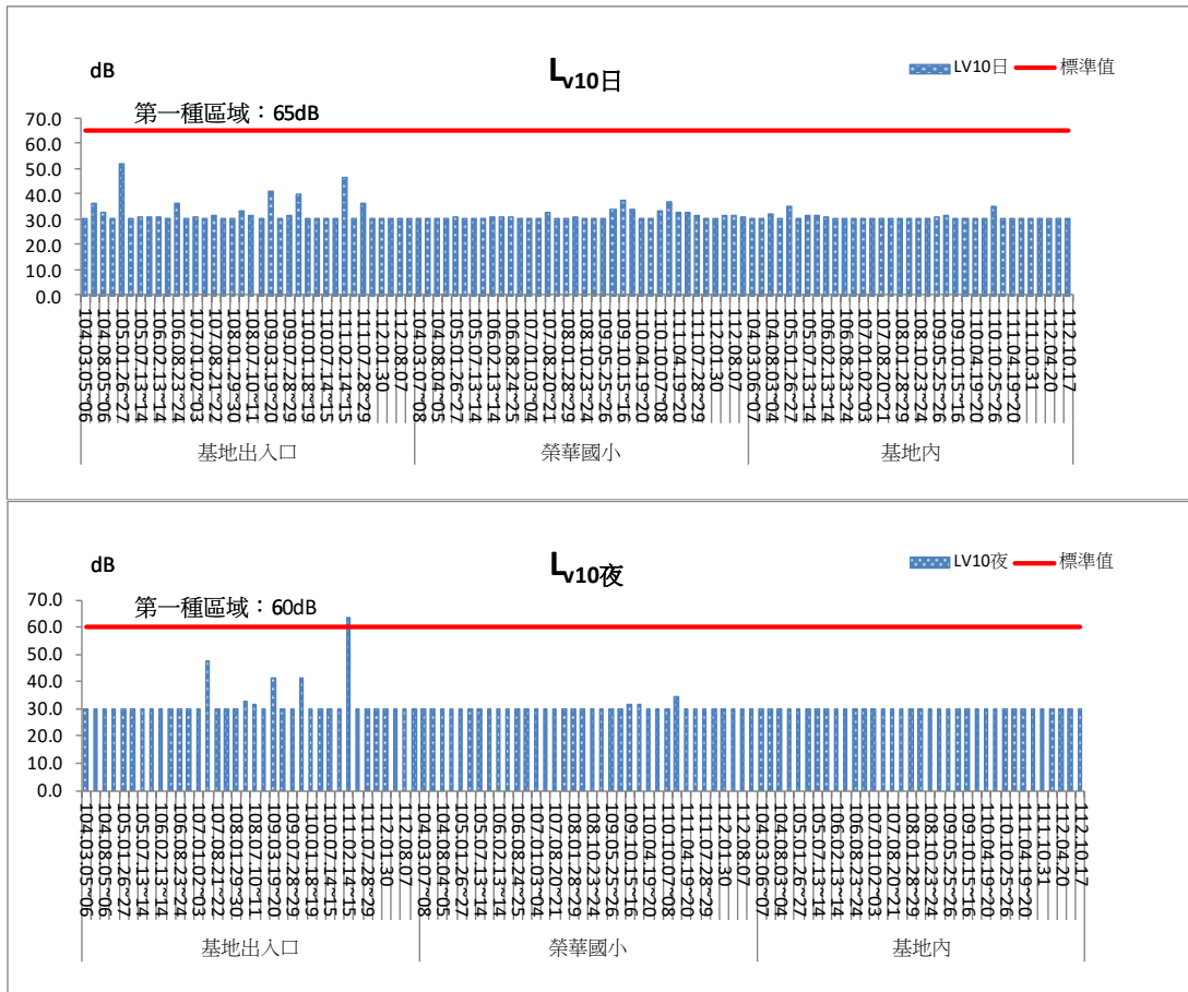
圖 2.2-3 基地出入口、榮華國小及基地內振動監測結果比較圖
