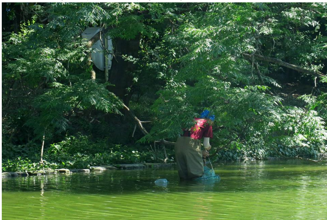
圖一、水域網具陷阱放置作業
