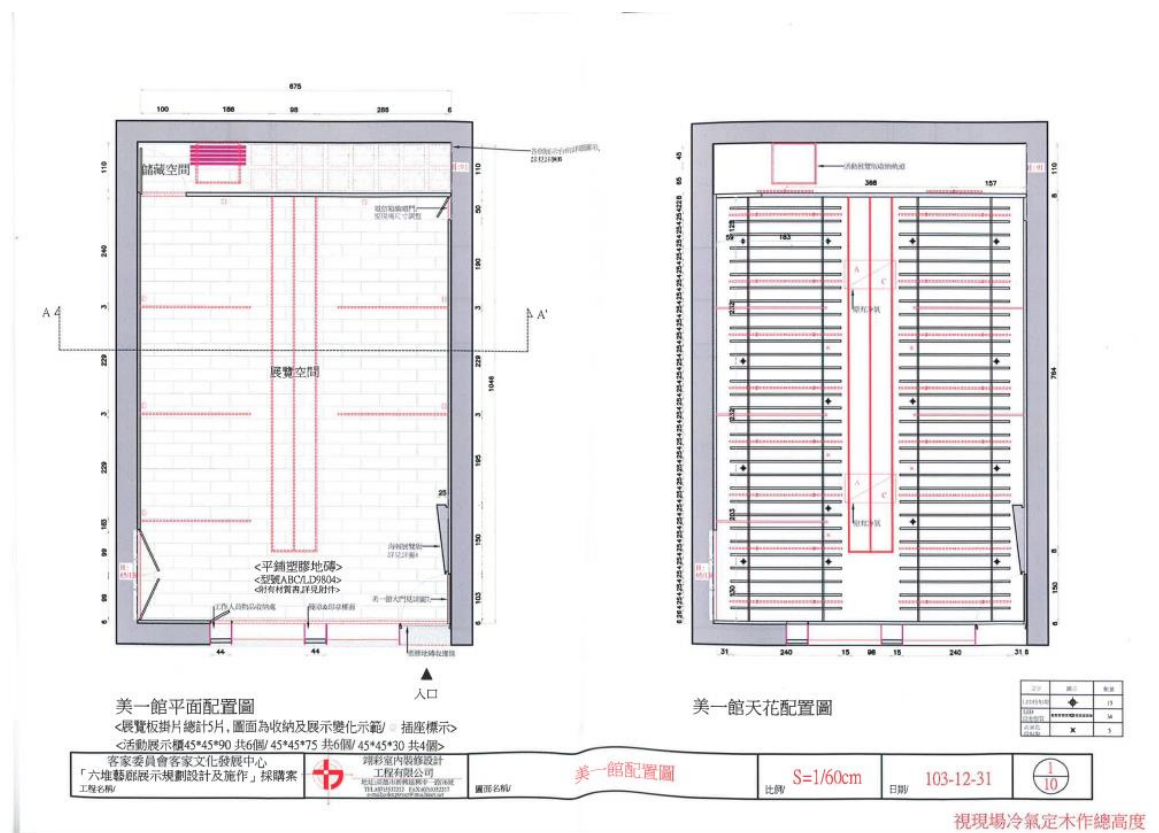
美一館平面圖
