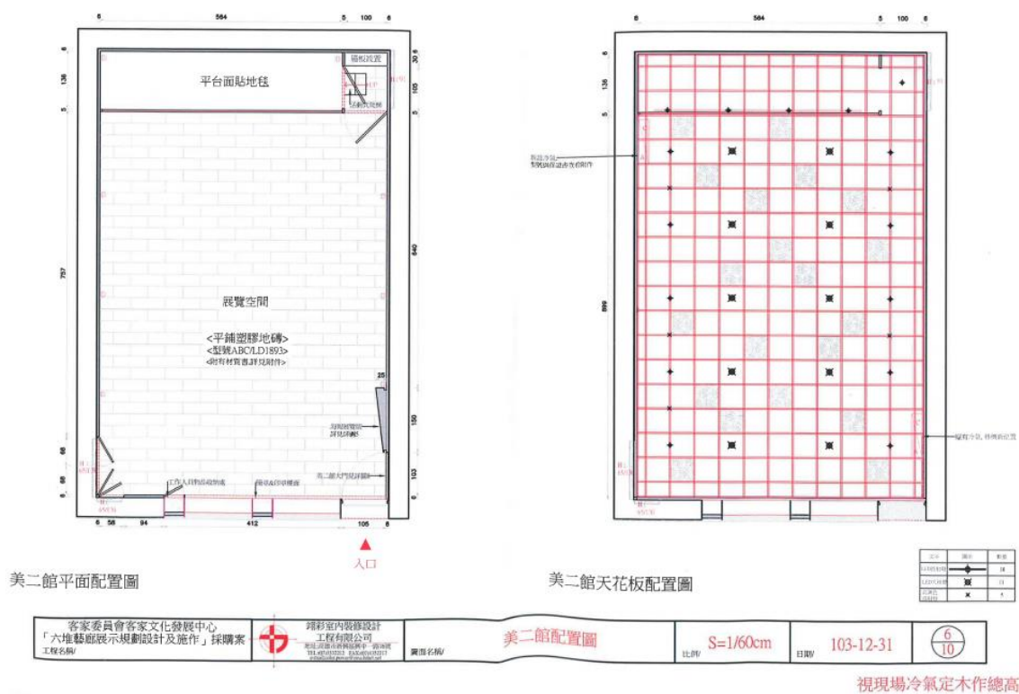
美二館平面圖
