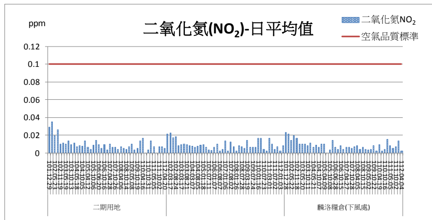
圖 2.1-7 二氧化氮各測點日平均值監測結果比較圖
