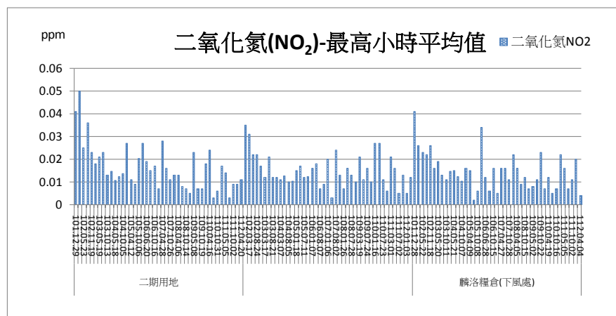
圖 2.1-8 二氧化氮各測點最高小時平均值監測結果比較圖
