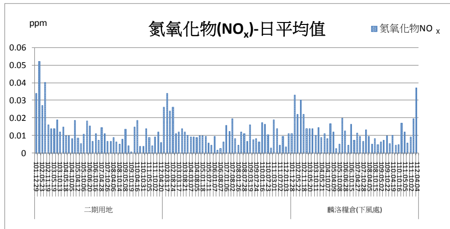
圖 2.1-10 氮氧化物各測點日平均值及監測結果比較圖
