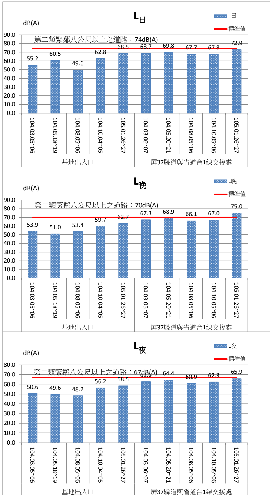
圖 2.2-1 基地出入口及屏 37 鄉道與台 1 省道交接處噪音監測結果比較圖
