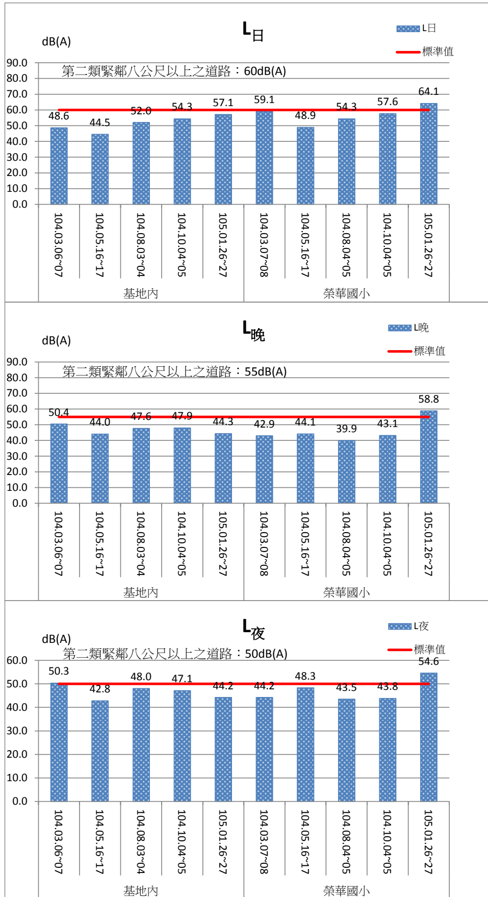
圖 2.2-2 基地內及榮華國小噪音監測結果比較圖
