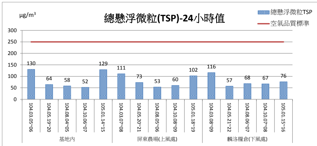
圖 2.1-1 TSP 各測點 24 小時監測結果比較圖
