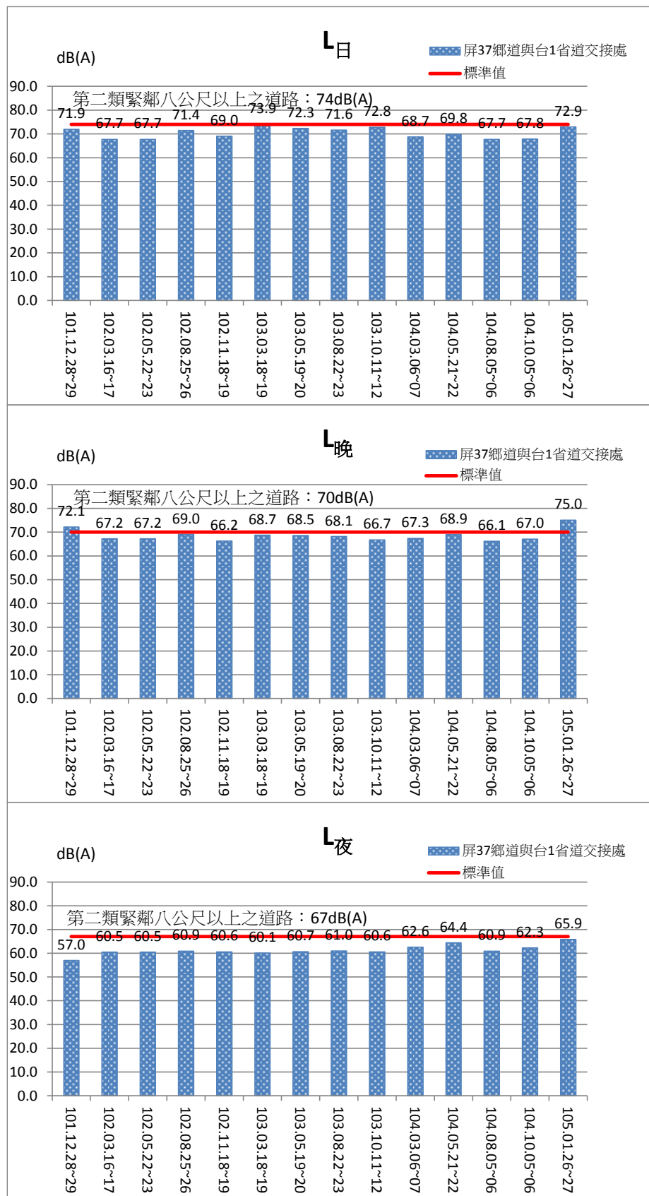
圖 2.2-2 屏 37 鄉道與台 1 省道交接處噪音監測結果比較圖
