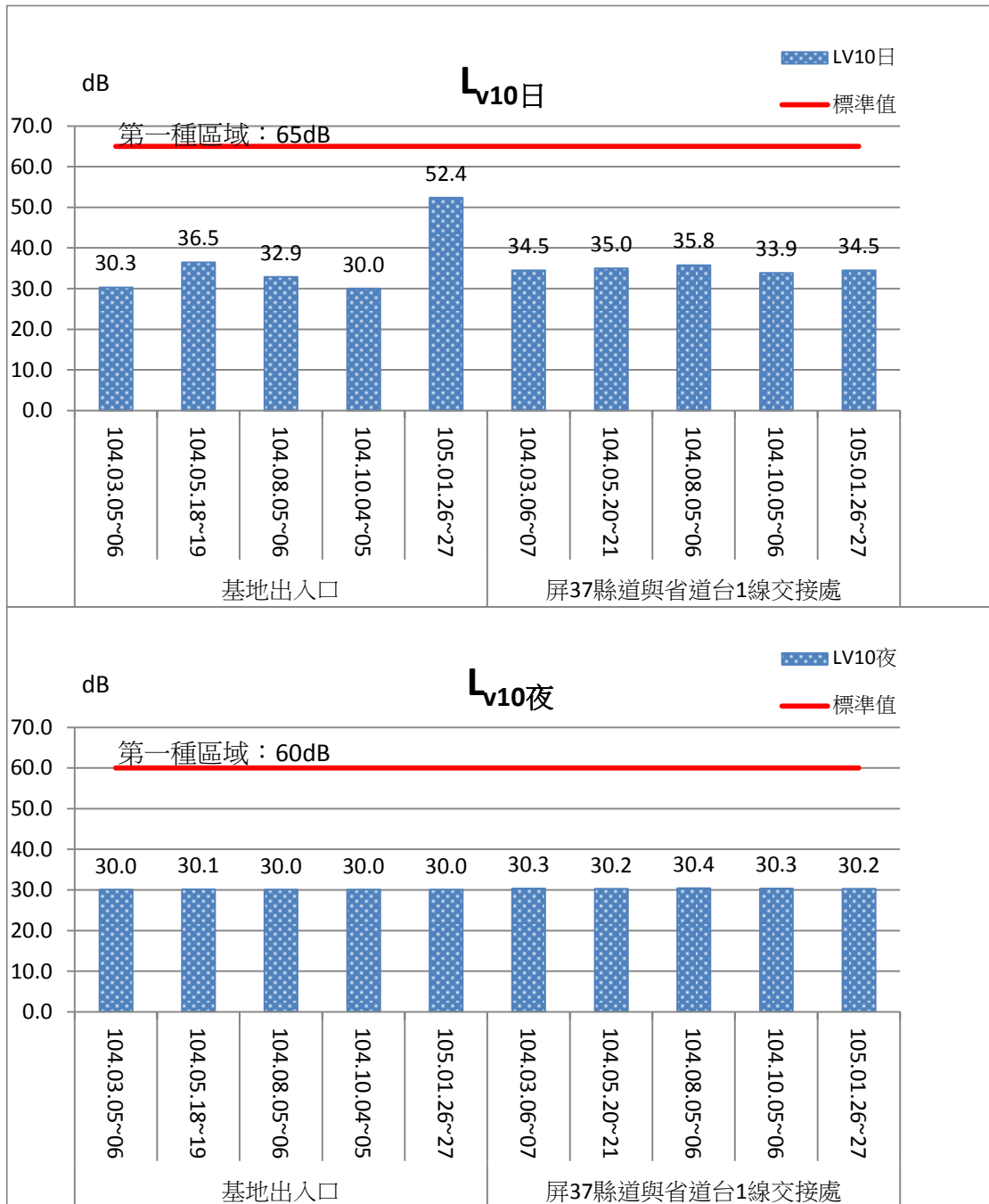
圖 2.2-3 基地出入口及屏 37 鄉道與台 1 省道交接處振動監測結果比較圖
