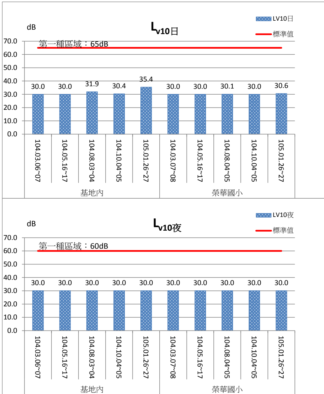
圖 2.2-4 基地內及榮華國小振動監測結果比較圖
