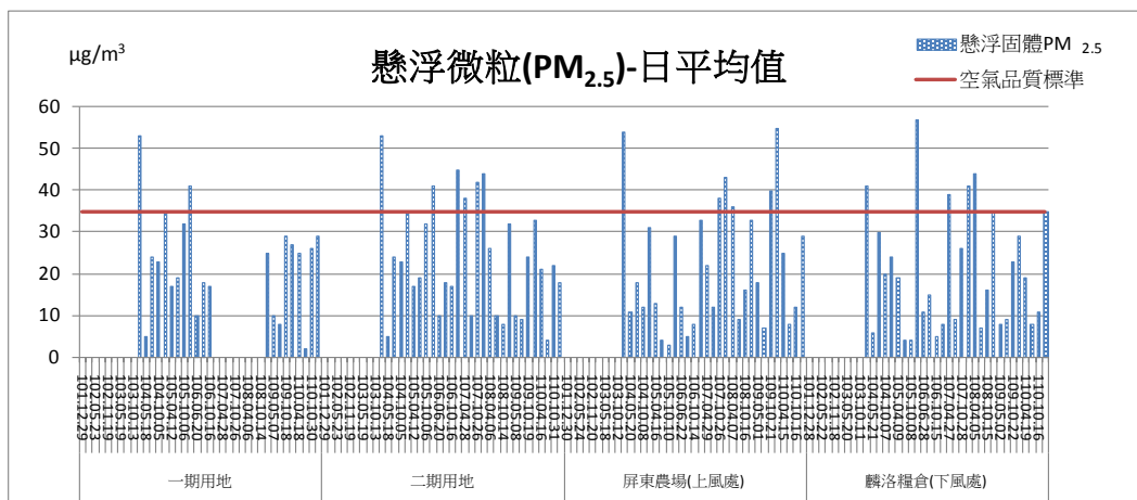
圖 2.1-15 PM 2.5 各測點日平均監測結果比較圖
