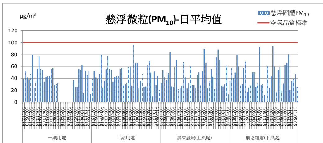
圖 2.1-2PM 10 各測點日平均值監測結果比較圖
