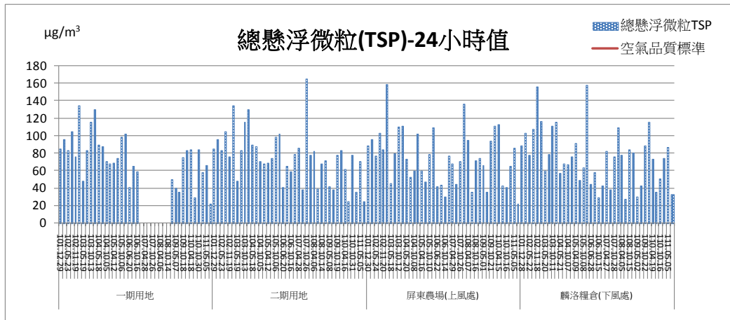
圖 2.1-1TSP 各測點 24 小時監測結果比較圖
