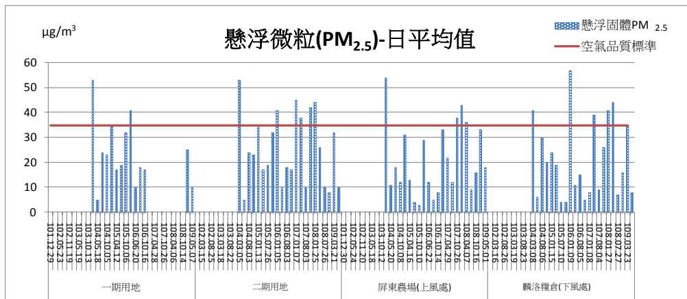
圖 2.1-15 PM 2.5 各測點日平均監測結果比較圖
